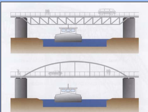
Die Tragwerkskonstruktion oberhalb der Fahrbahn schafft die erforderliche Durchfahrthöhe von mindestens 5,25 m, ohne die Fahrbahn unnötig hoch anzuheben
